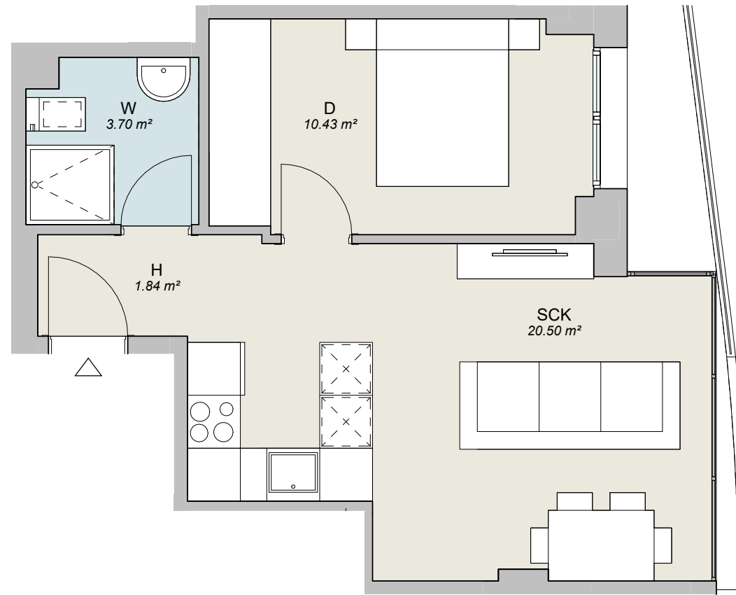
VIV.B PORTAL 1-P.01-VIV.B 1:60
